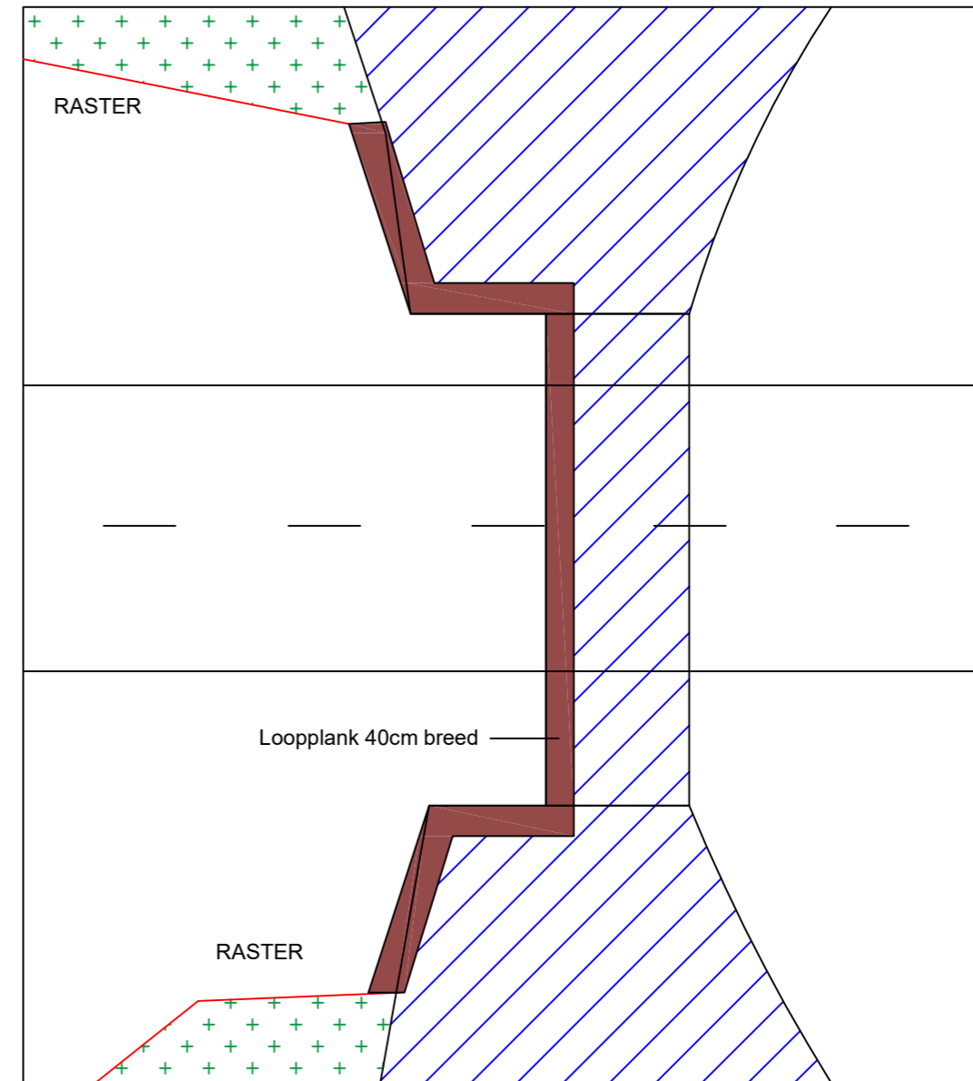
BOVENAANZICHT PRINCIPE
